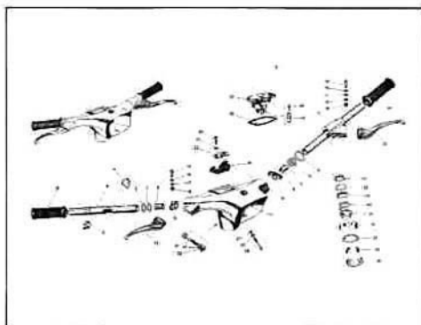
GRUPO DIRECCION - MANILLAR
