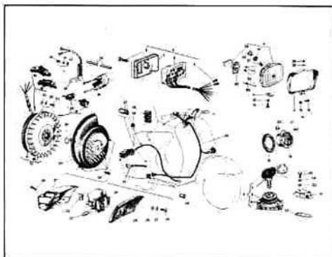
GRUPO ELECTRICO
