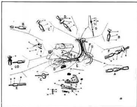
GRUPO TRANSMISIONES
